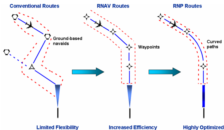
Figura 3.8: Rutas convencionales, RNAV y RNP [Fig11].
