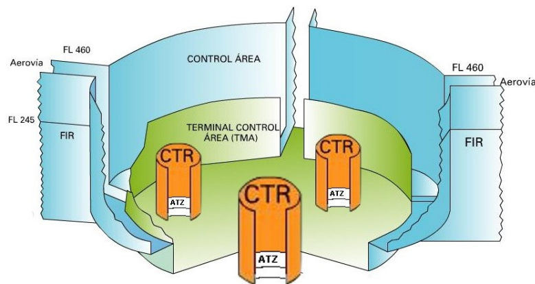
Figura 3.11: Sectorización de las zonas de control ATC [Fig15].
