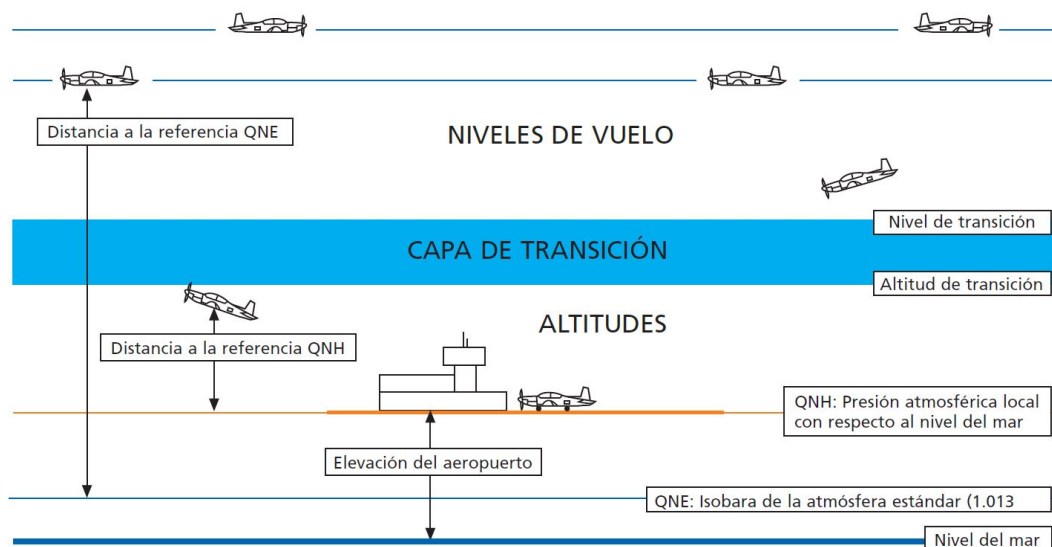
Figura 3.17: Altimetría en navegación aérea [6].
