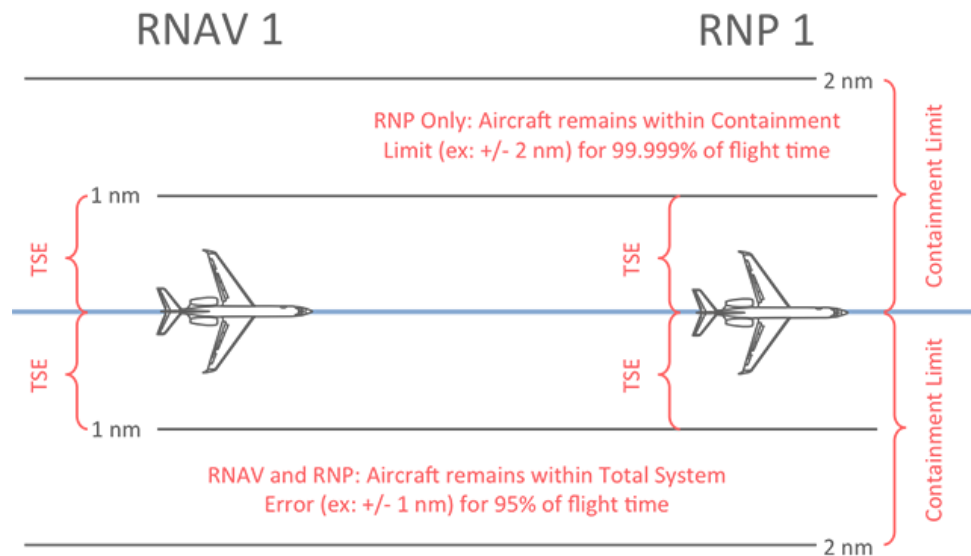
Figura 3.9: Diferencias y similitudes entre RNAV y RNP [Fig12].
